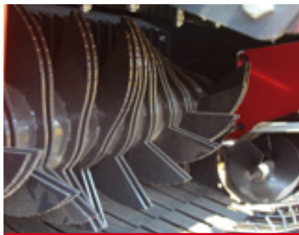
Infaldatore con rotore. / Rotor feeding system. / Alimentador simple con rotor. / Plieuse à rotor.
